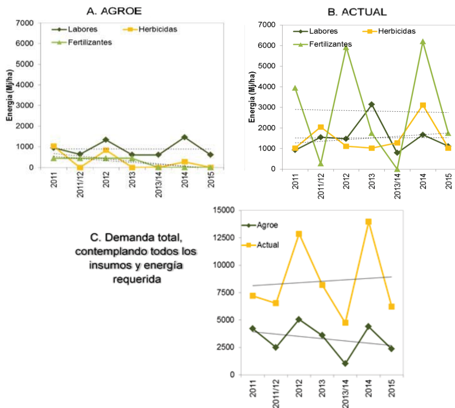
Figura 5. Evolución de la demanda de energía, según principales insumos En líneas punteadas se muestran las tendencias.
